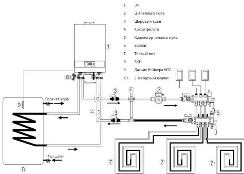
Рис. 20. Схема подключения «ЭЖ + БКН + Теплый пол».
