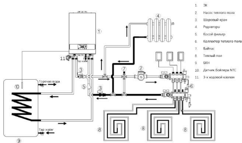
Рис. 21. Схема подключения «ЭЖ + БКН + Теплый пол + Радиаторы».
